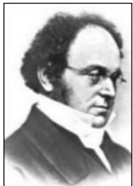
Augustus De Morgan 1806 - 1871
