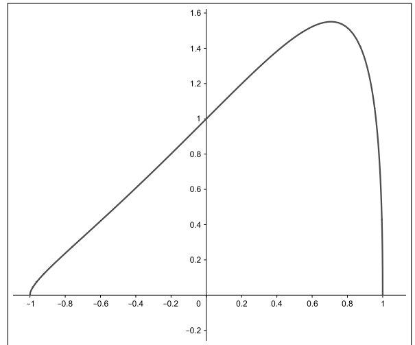
Γραφική παράσταση της συνάρτησης
